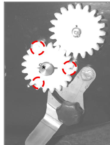
Рис. 1:Вытащите шплинт!
