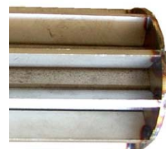
Высевной вал для посева трав (пшеница)
